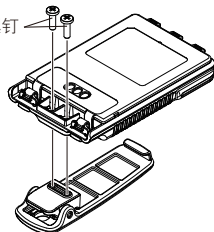
① 将快速释放皮套的底部插片插入 FT5DR 底部的槽中
